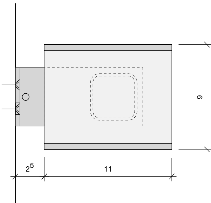
Grundriss
