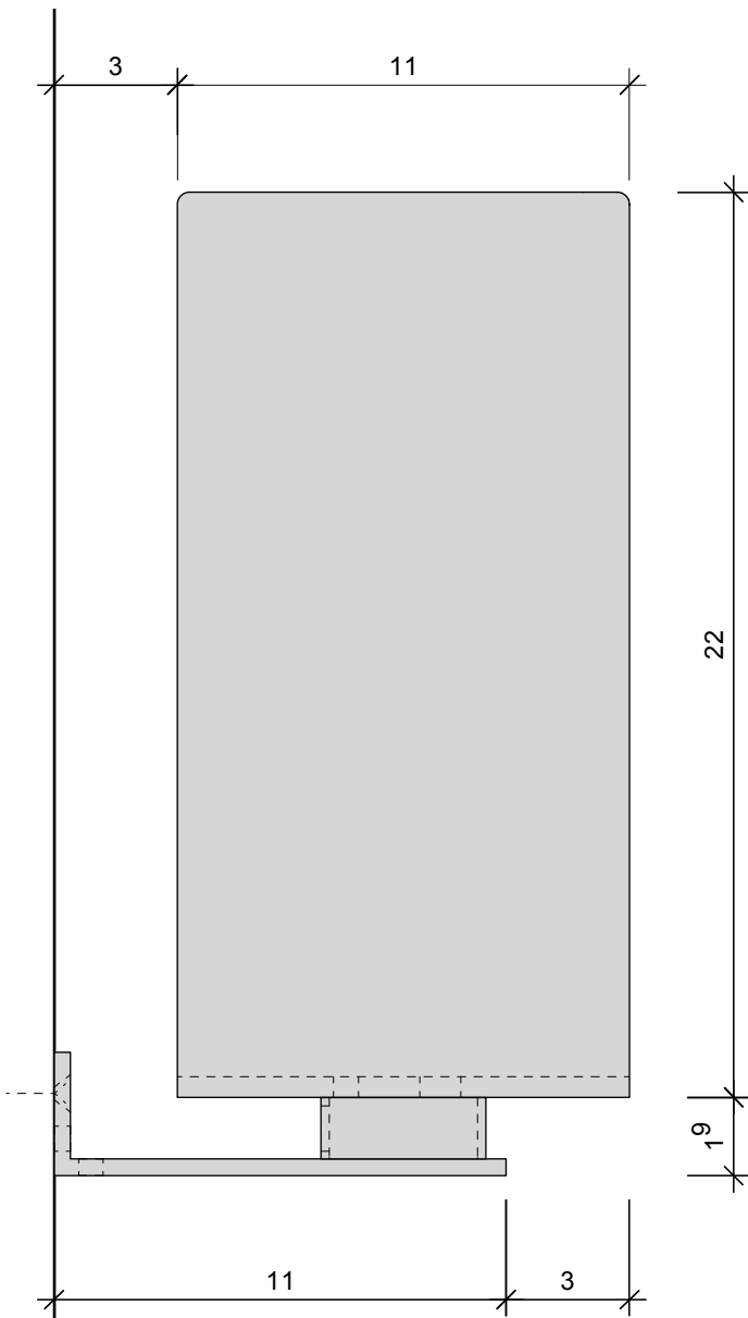
Seitenansicht
